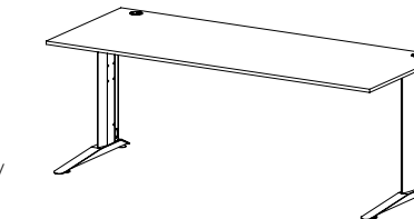
VA 85 stůl pracovní / 2000 x 750 x 800 /
