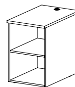
VA 27 stůl pod tiskárnu / 500 x 750 x 800 /
