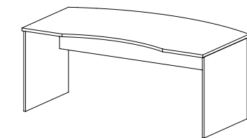
VA 80 stůl pracovní tvarový / 1800 x 750 x 1000/800 /
