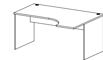
VA 79 stůl pracovní tvarový / 1600 x 750 x 1200/400 /
