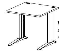
VA 49 stůl pracovní / 1600 x 750 x 800 /
