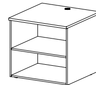
VA 26 stůl pod tiskárnu / 800 x 750 x 800 /
