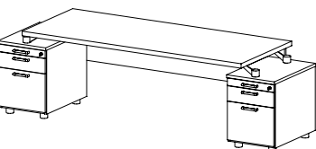
EX 90 stůl pracovní rovný (kontejner EX 109) / 2524 x 730 x 800 /
