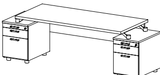
EX 82 stůl pracovní rovný (kovové nohy) / 2324 x 730 x 800 /
