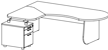
EX 62P stůl pracovní tvarový (kovové nohy) / 2250 x 730 x 1912 /
