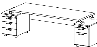
EX 91 stůl pracovní rovný (kontejner EX 108, 109) / 2524 x 730 x 800 /
