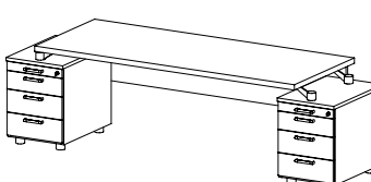
EX 89 stůl pracovní rovný (kontejner EX 108) / 2524 x 730 x 800 /
