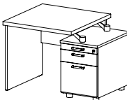
EX 67P stůl pracovní rovný (kovové nohy) / 1062 x 730 x 800 /
