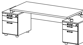
EX 74 stůl pracovní rovný (kovové nohy) / 2124 x 730 x 800 /
