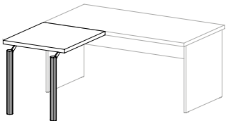
EX 93 boční přídavný stůl (kovové nohy) / 874 x 730 x 700 /
