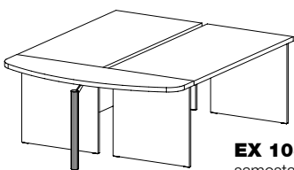
EX 101 samostatná stolová clona pro stolové sestavy / 1210 x 350 x 19 /
