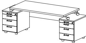
EX 73 stůl pracovní rovný (kovové nohy) / 2124 x 730 x 800 /
