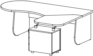
EX 58P stůl pracovní tvarový (kovové nohy) / 2250 x 730 x 1912 /
