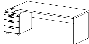
EX 77L stůl pracovní rovný (kovové nohy) / 2062 x 730 x 800 /
