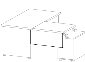
EX 99 samostatná stolová clona pro EX 92 / 830 x 350 x 19 /
