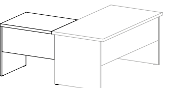
EX 94P boční přídavný stůl / 800 x 730 x 700 /
