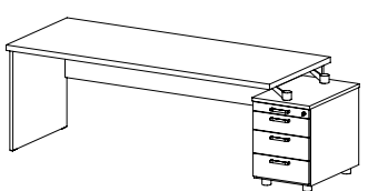
EX 87P stůl pracovní rovný (kontejner EX 108) / 2262 x 730 x 800 /
