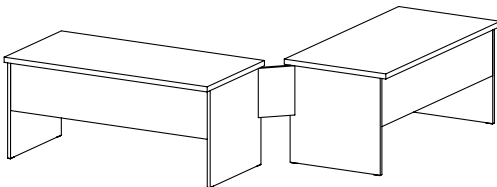
EX 102 samostatná stolová clona pro stolové sestavy / 261 x 350 x 19 /
