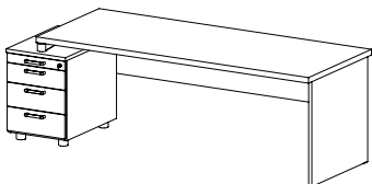
EX 85L stůl pracovní rovný (kontejner EX 108) / 2262 x 730 x 800 /
