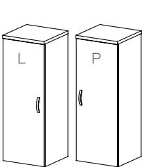
ST 08 L/P skříňka policová s dveřmi / 400 x 1100 x 400 /
