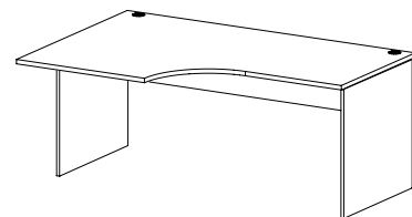
ST 76 stůl pracovní tvarový / 1800 x 750 x 1200/800 /
