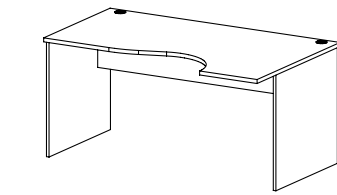
ST 75 stůl pracovní tvarový / 1600 x 750 x 1000/400 /
