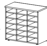
ST 110 skříň registrační / 800 x 1100 x 400 /
