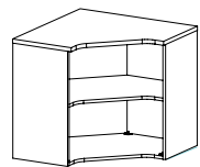
ST 116 skříň rohová / 800 x 1100 x 800 /
