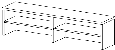
ST 34 pultová nástavba / 1400 x 350 x 320 /
