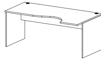
ST 73 stůl pracovní tvarový / 1800 x 750 x 1000/400 /
