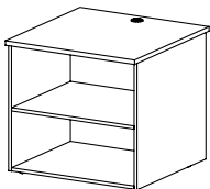
ST 26 stůl pod tiskárnu / 800 x 750 x 800 /
