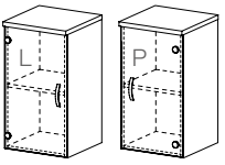
ST 12 L/P skříňka policová se skleněnými dveřmi / 400 x 750 x 400 /
