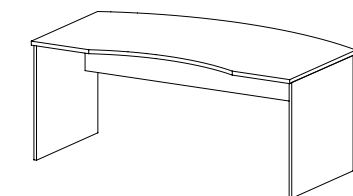
ST 80 stůl pracovní tvarový / 1800 x 750 x 1000/800 /
