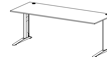
ST 84 stůl pracovní s kovovou podnoží / 1800 x 750 x 800 /
