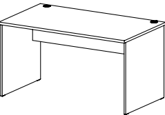
ST 28 stůl pracovní / 1400 x 750 x 800 /
