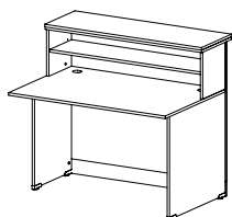
RE 07/18 RE 07/25 recepce rovná levá / 1200 x 1100 x 880 /
