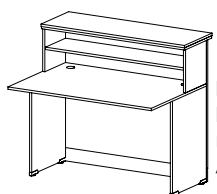
RE 07/18 RE 07/25 recepce rovná levá / 1200 x 1100 x 880 /
