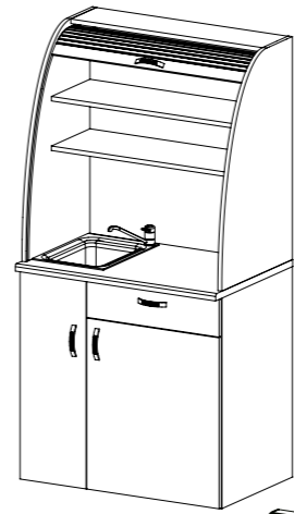
KU 90ROL2 minikuchyňka s dřezem a vodovodní baterií / 900 x 1800 x 650 /
