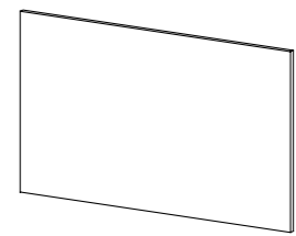
KU 70 obkladová deska rozměry obkladových desek KU 70/900 / 900 x 18 x 500 / KU 70/1200 / 1200 x 18 x 500 / KU 70/1500 / 1500 x 18 x 500 / KU 70/1800 / 1800 x 18 x 500 / KU 70/2100 / 2100 x 18 x 500 / KU 70/2400 / 2400 x 18 x 500 / KU 70/2700 / 2700 x 18 x 500 /
