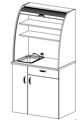
KU 90ROL4 minikuchyňka s dřezem, vodovodní baterií a lednicí / 900 x 1800 x 650 /
