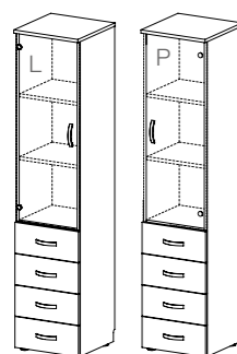
BASIC 02-13 L/P Skříň policová se skleněnými dveřmi a 4 dřevěnými zásuvkami / 400 x 1800 x 400 /
