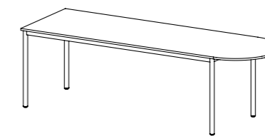
BASIC 51 D Stůl koncový – psací i jednací s kovovou podnoží / 2400 x 745 x 800 /
