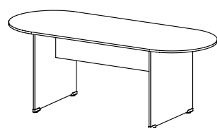
BASIC 58 A Stůl jednací – ovál / 2000 x 745 x 800 /
