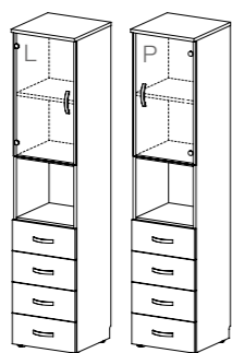
BASIC 02-11 L/P Skříň policová se skleněnými dveřmi a 4 dřevěnými zásuvkami / 400 x 1800 x 400 /
