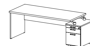
EX 80P stůl pracovní rovný (kontejner EX 109) / 2062 x 730 x 800 /
