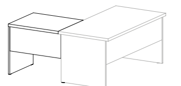
EX 94P boční přídavný stůl / 800 x 730 x 700 /
