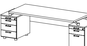
EX 83 stůl pracovní rovný (kontejner EX 108, 109) / 2324 x 730 x 800 /
