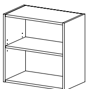
KUH 60 kuchyňská skříňka horní bez dvířek / 600 x 600 x 280 /
