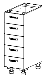
KU 30 Z5 kuchyňská skříňka zásuvková / 300 x 824 x 528 /
