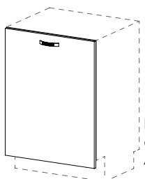
KU 63 dvířka na myčku / 596 x 720 x 18 /
