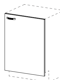
KU 64P dvířka na lednici, pravé / 596 x 720 x 18 /
