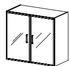
DE 42 nástavec nízký s proskl. dveřmi / 900 x 800 x 450 /
