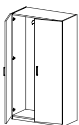
DE 21 skříň šatní střední s dveřmi / 900 x 1640 x 450 /
