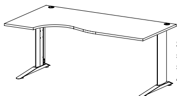
ST 60 stůl pracovní tvarový s kovovou podnoží / 1800 x 750 x 1000/400 /
