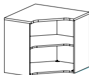
ST 116 skříň rohová / 800 x 1100 x 800 /
