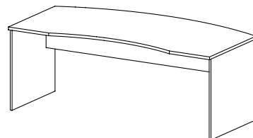
ST 81 stůl pracovní tvarový / 2000 x 750 x 1000/800 /
