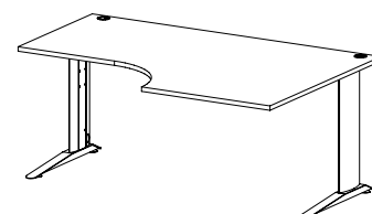
ST 65 stůl pracovní tvarový s kovovou podnoží / 1800 x 750 x 1200/800 /
